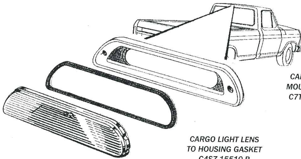
CARGO LIGHT LENS C4SZ-15514-B
